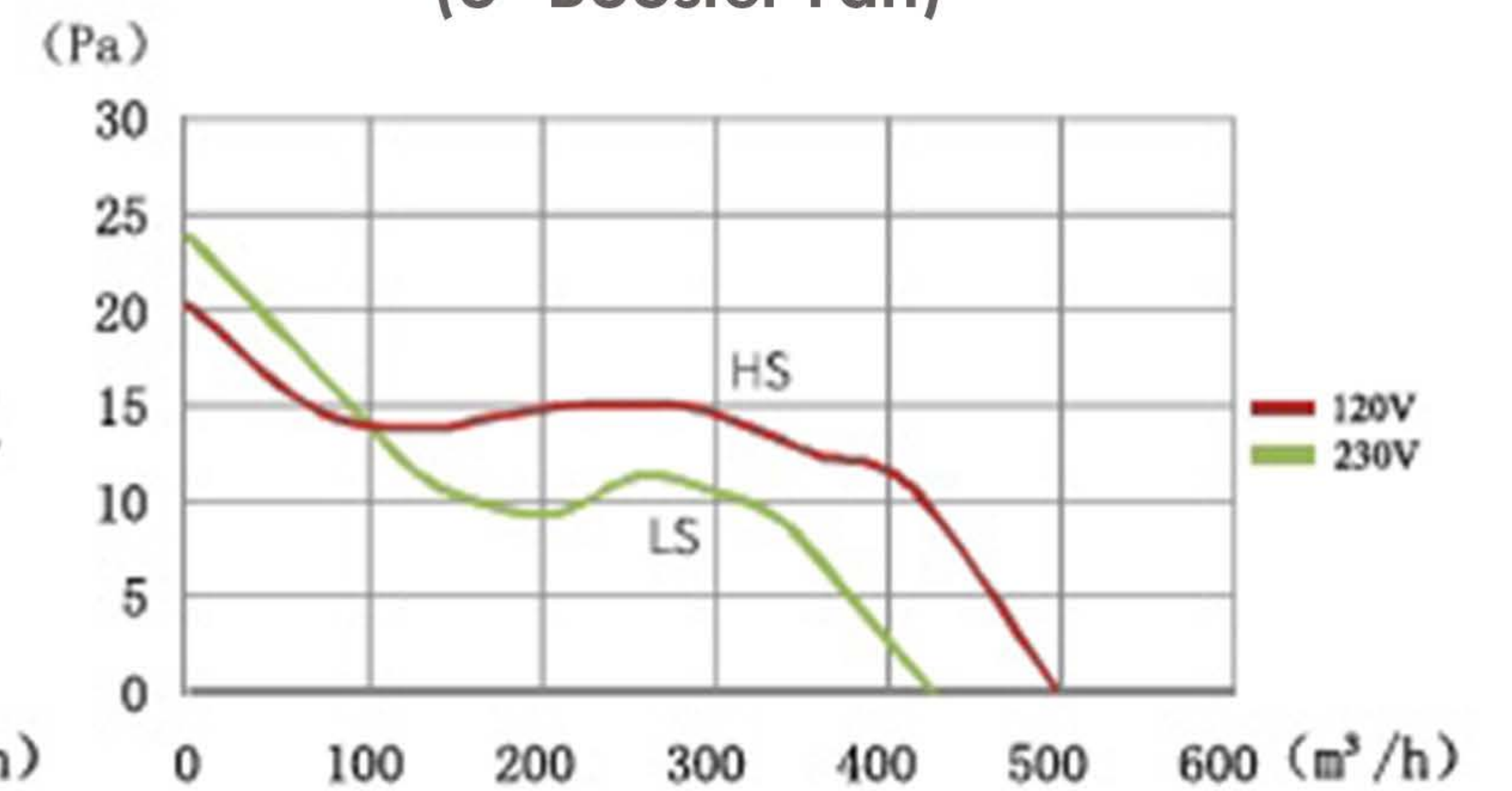
HI-200IS (8" Booster Fan)
