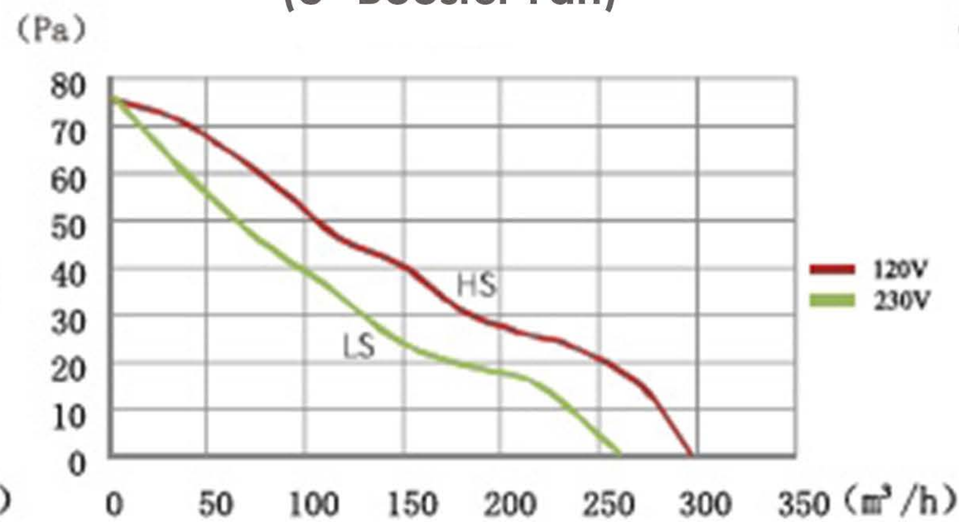
HI-150IS (6" Booster Fan)
